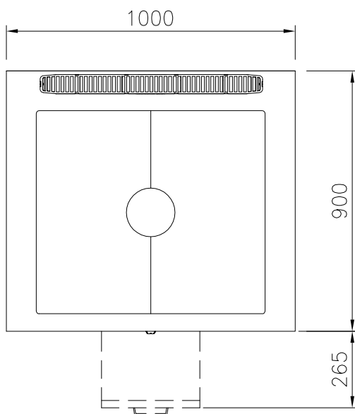
Boven aanzicht
